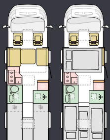
670 DL
