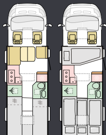
650 DL
